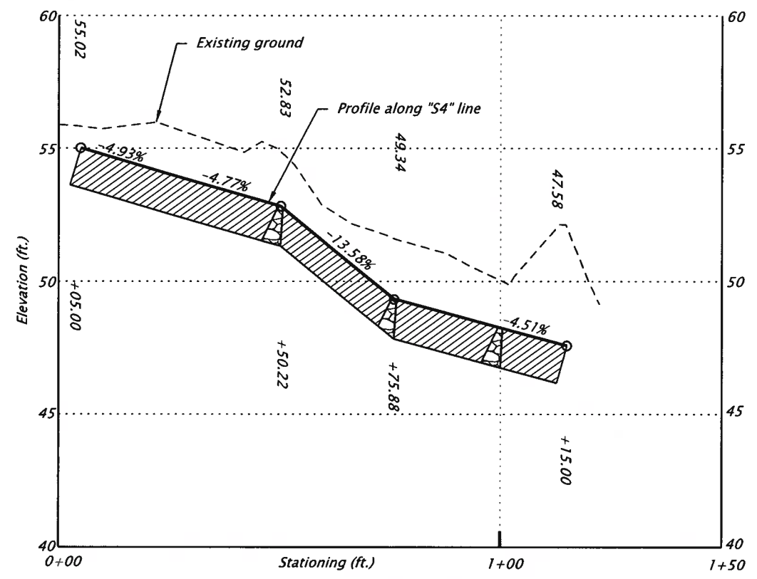
PROFILE "S4" LINE Horiz. Scale: 1" = 30' Vert. Scale: 1" = 5'
